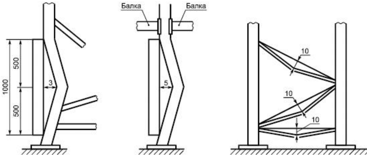
Рисунок Б.1 - Максимальные допустимые значения деформации элементов
